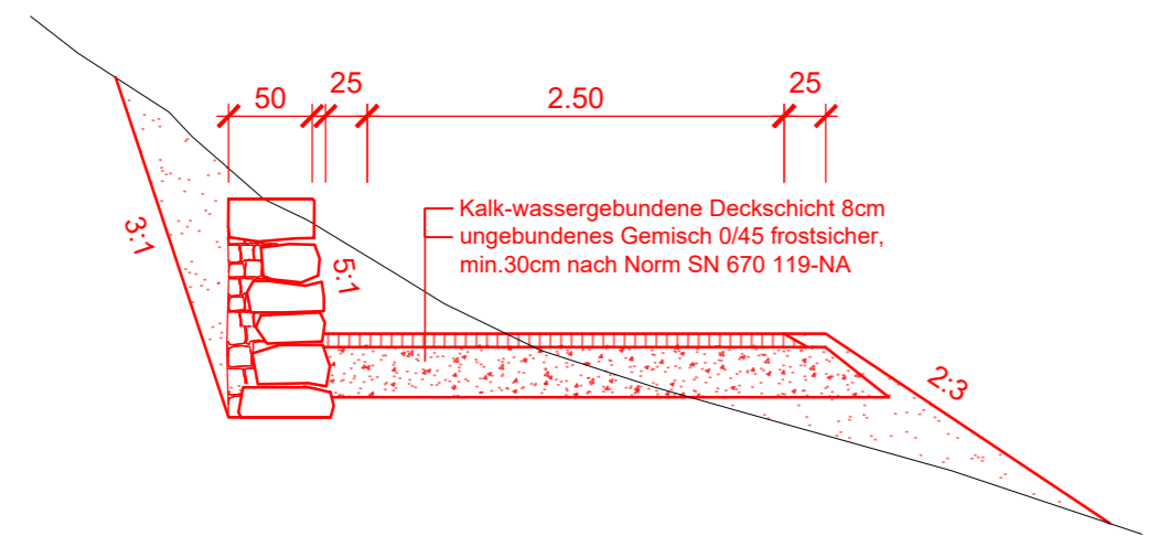
Normalprofil 1:50 Bergseitige Trockensteinmauer
