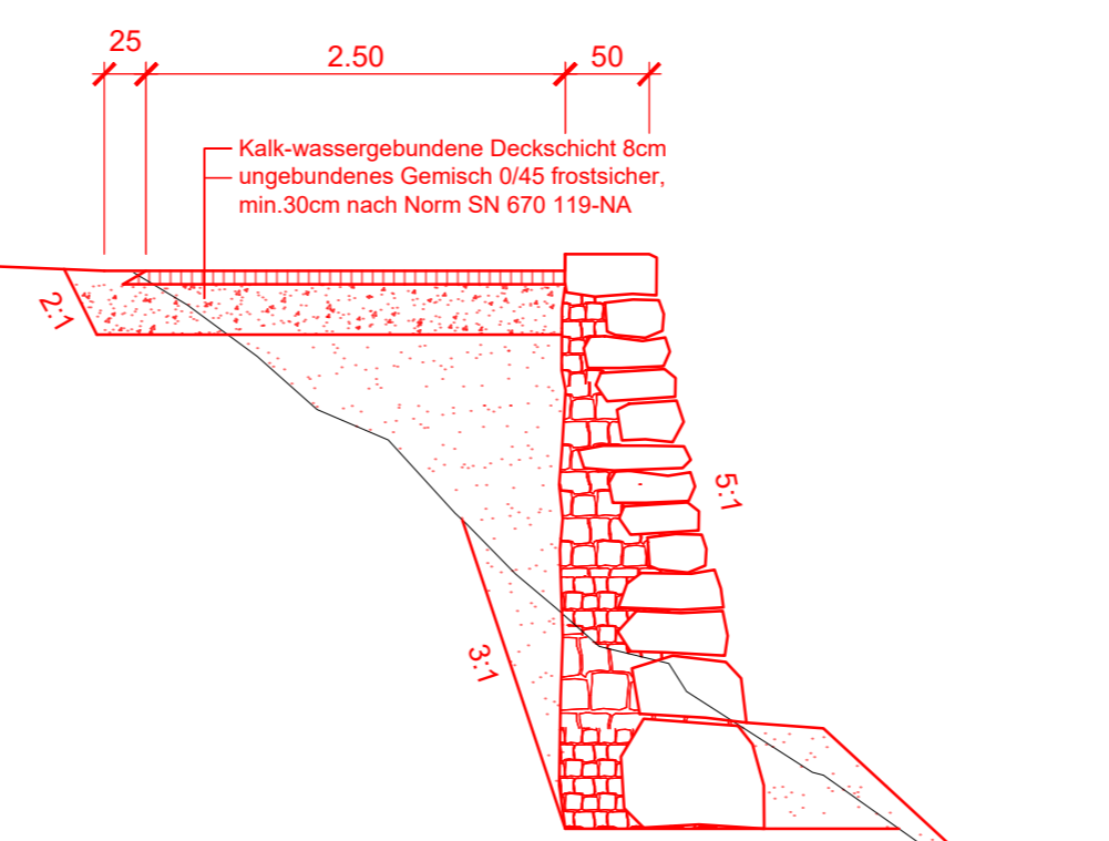
Normalprofil 1:50 Talseitige Trockensteinmauer
